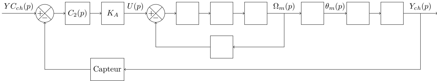
Figure A Modèle de la commande du chariot
