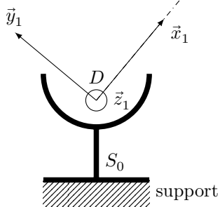
Figure A Schéma cinématique plan d'un axe motorisé (réponses aux questions 1 et 2)
